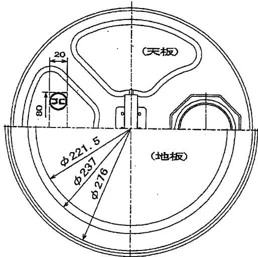
UNマーク表示位置(B)
